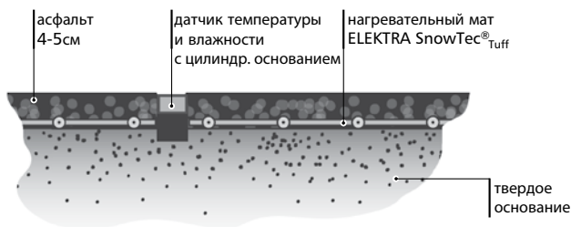
Поперечное сечение дороги с асфальтобетонным покрытием
